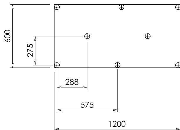
Grid-3 para placa recortada com 600 x 1200
