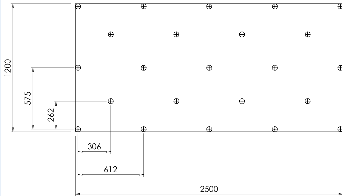
Grid-1 para painel wall com 1200 x 2500 (Dimensão Padrão)
