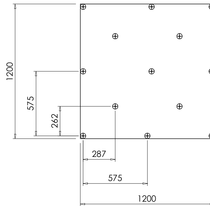
Grid-2 para placa recortada com 1200 x 1200
