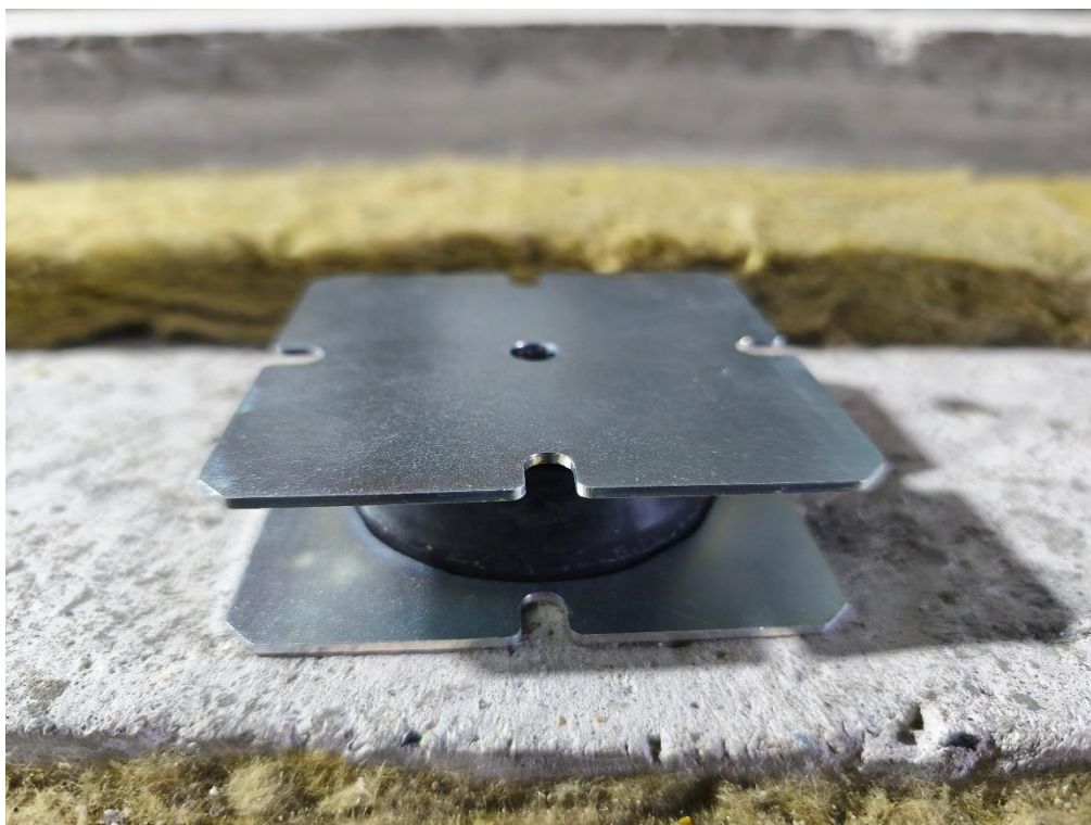
Foto A.1: Detalhe da amostra ensaiada.
