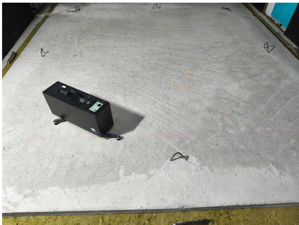
Foto A.3: Ensaio com a máquina de impacto.
