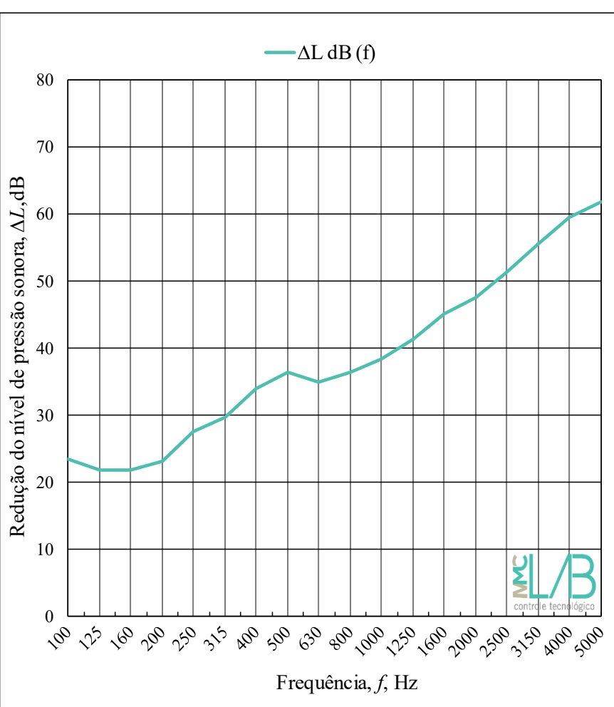
Figura 4.2- Redução do nível de pressão sonora ( \Delta L ) em bandas de terço de oitava.
