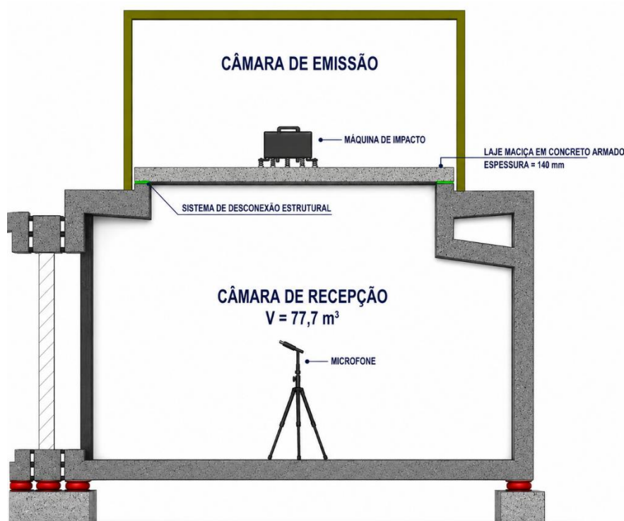
Figura 3.1- Corte da câmara onde foram realizadas as medições.
