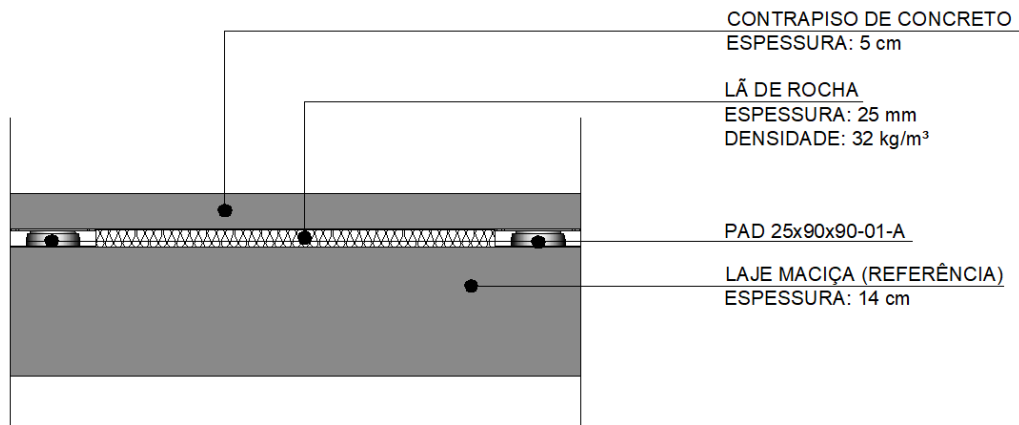
Figura 2.1- Representação esquemática da amostra ensaiada.
