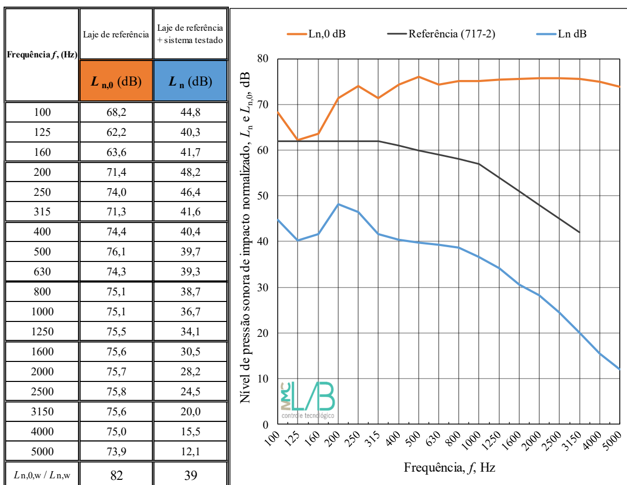
Figura 4.1- Valores de nível de pressão sonora de impacto normalizado ( L_n e L_{n,0} ).
